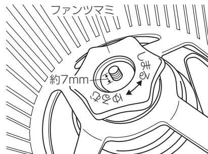
【正規位置でファンツマミを締め込んだ状態】
